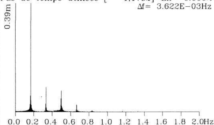
Sonde de dénivellation 3
